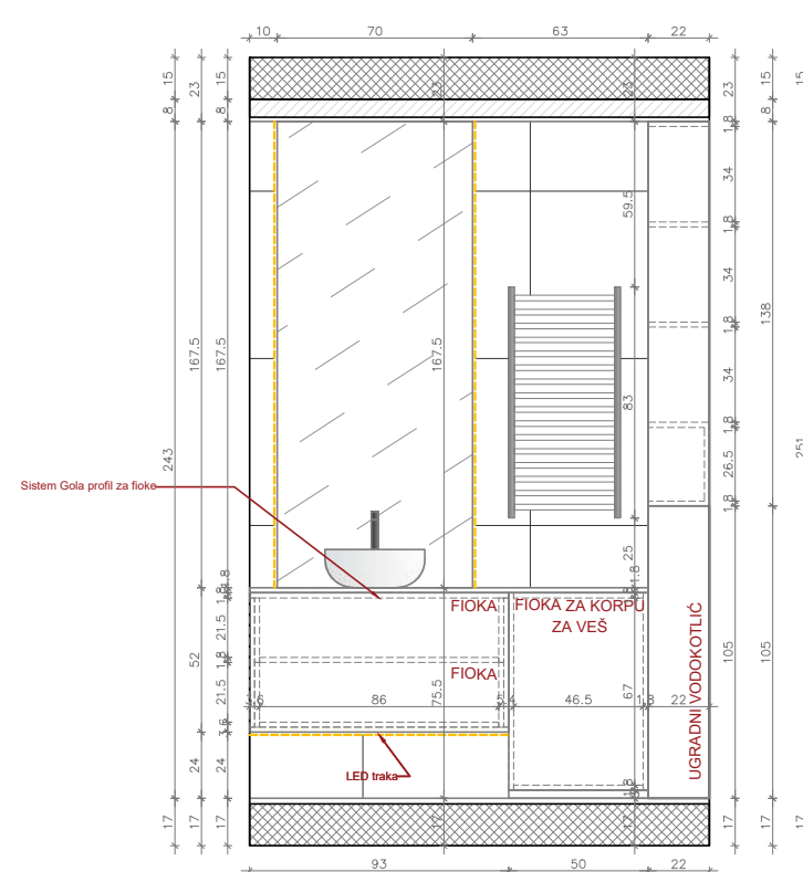
L – PRESEK NAEŠTAJA U KUPATILU
