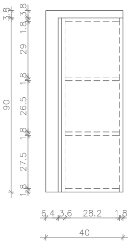
K – IZGLED ŠANK
