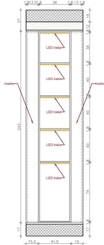
P6 – IZGLED POLICE U DEČIJOJ SOBI
