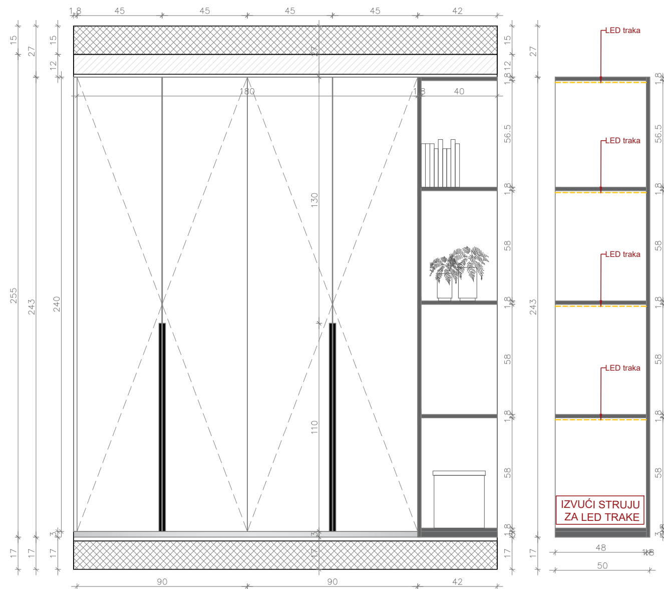
P4 – OSNOVA PLAKARA U DEČIJOJ SOBI
