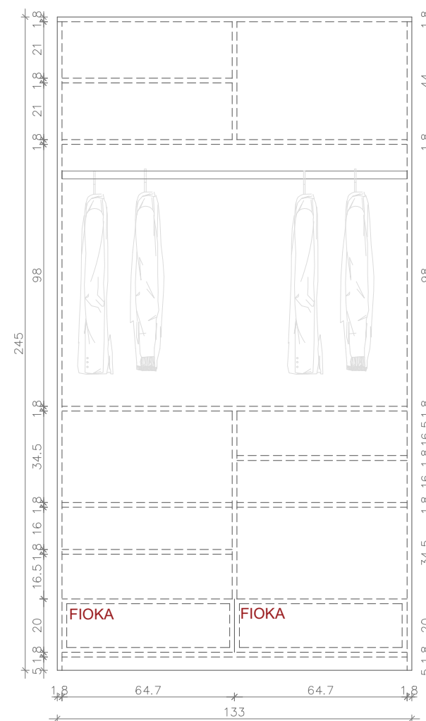
P2 – PRESEK ORMARA
