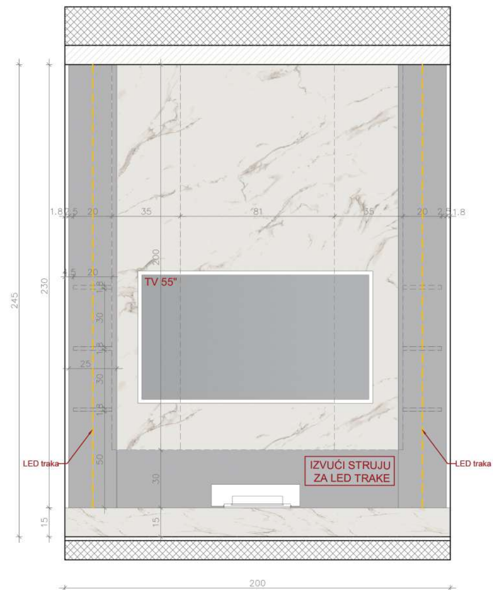
TV – IZGLED TV ZIDA
