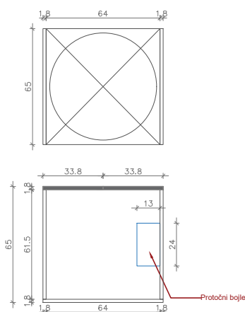
M – OSNOVA NAMEŠTAJA U KUPATILU
