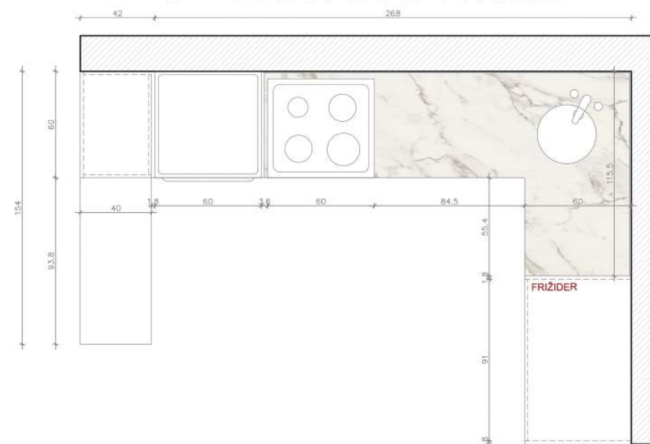
K — OSNOVA RADNE POVRŠINE
