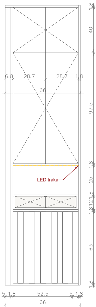
P1 – IZGLED ORMARA
