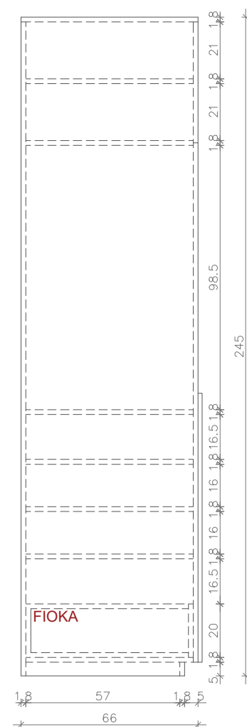
P2 – OSNOVA ORMARA
