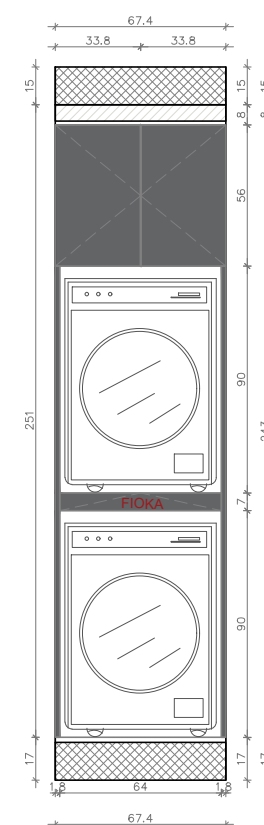
M – IZGLED ZIDA U KUPATILU
