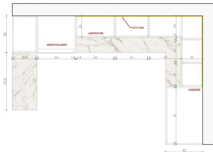
K — OSNOVA GORNJIH ELEMENATA
