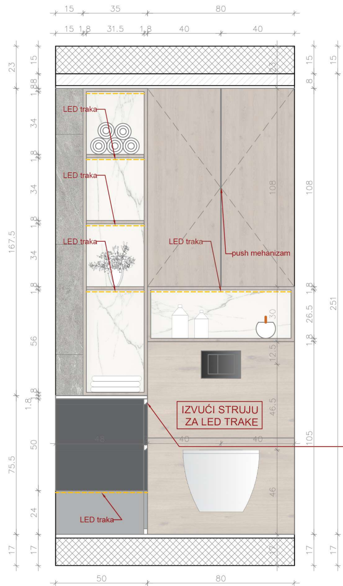
W – IZGLED ZIDA U KUPATILU
