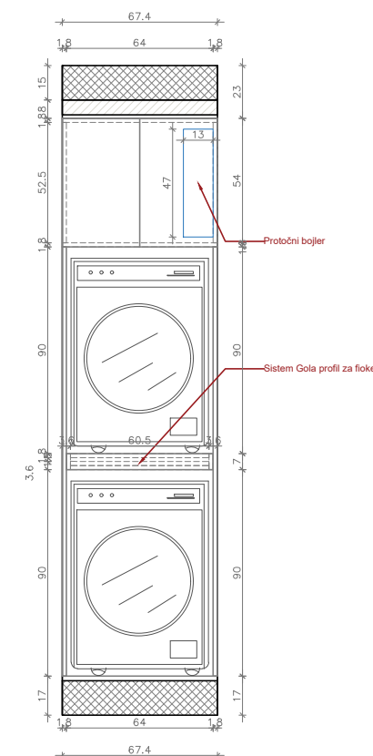
M – OSNOVA NAMEŠTAJA U KUPATILU
