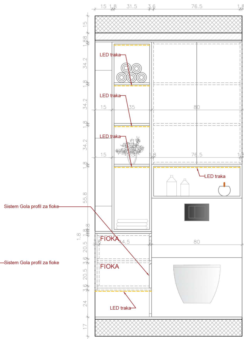
W – PRESEK NAMEŠTAJA U KUPATILU
