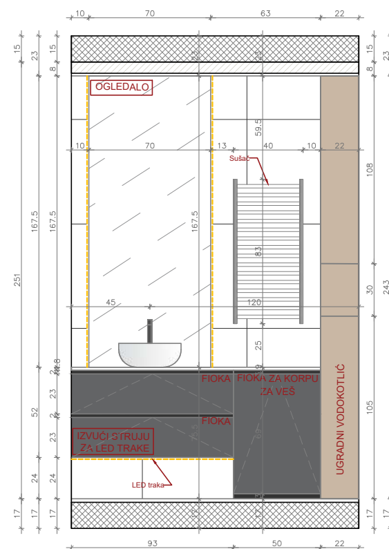
L – IZGLED ZIDA U KUPATILU
