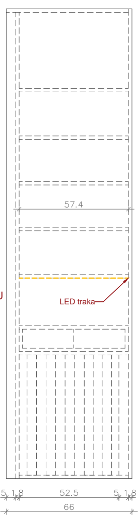
P1 – PRESEK ORMARA
