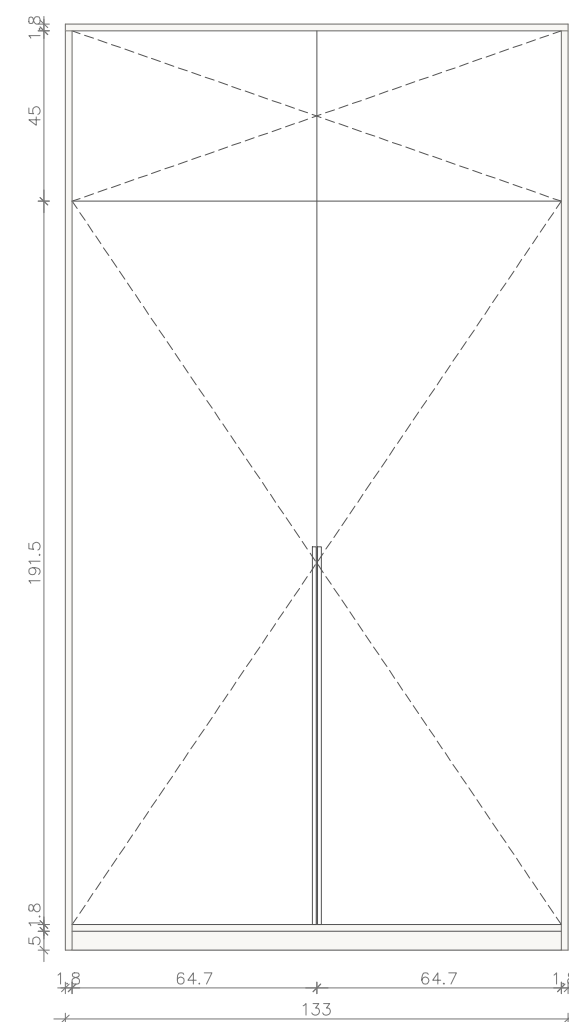
P2 – IZGLED ORMARA
